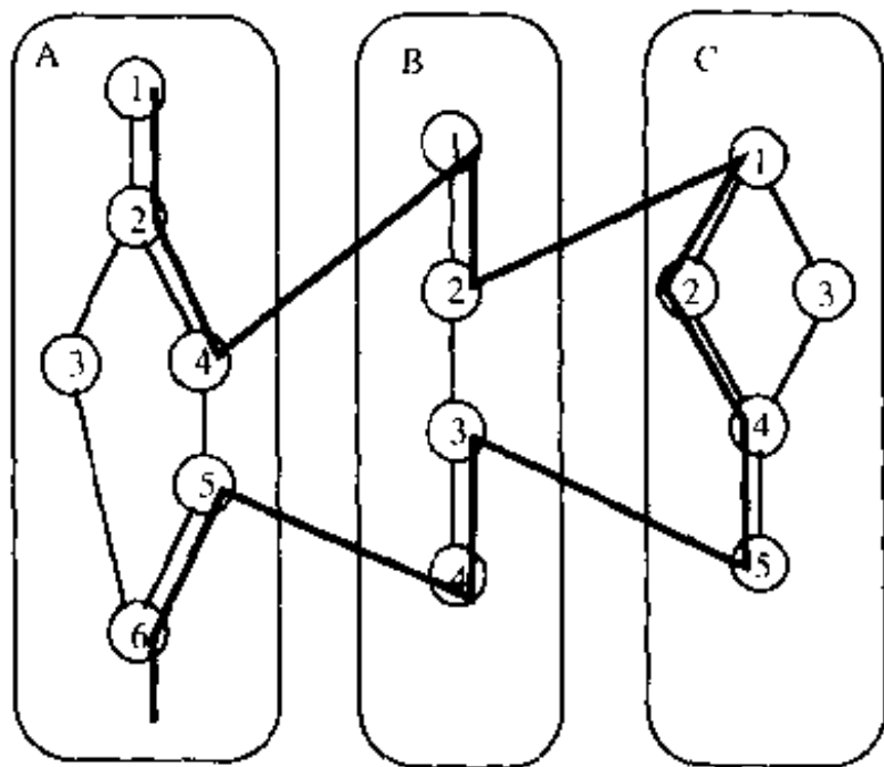
图13-8 跨三个单元的MM-路径
