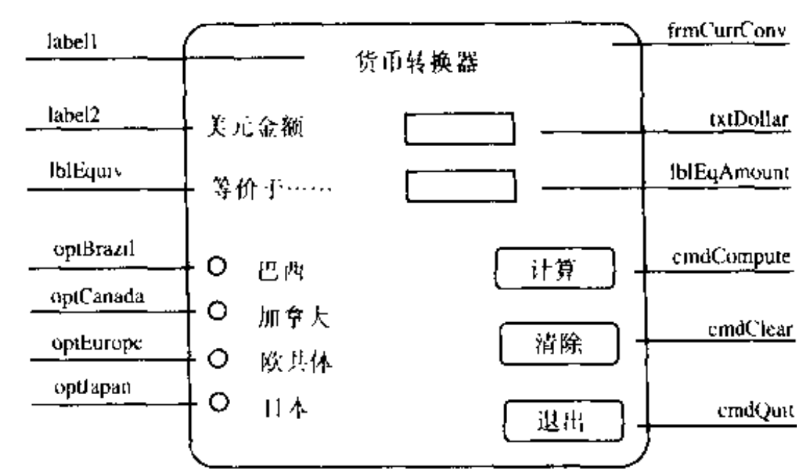
图20-2 Visual Basic控件
