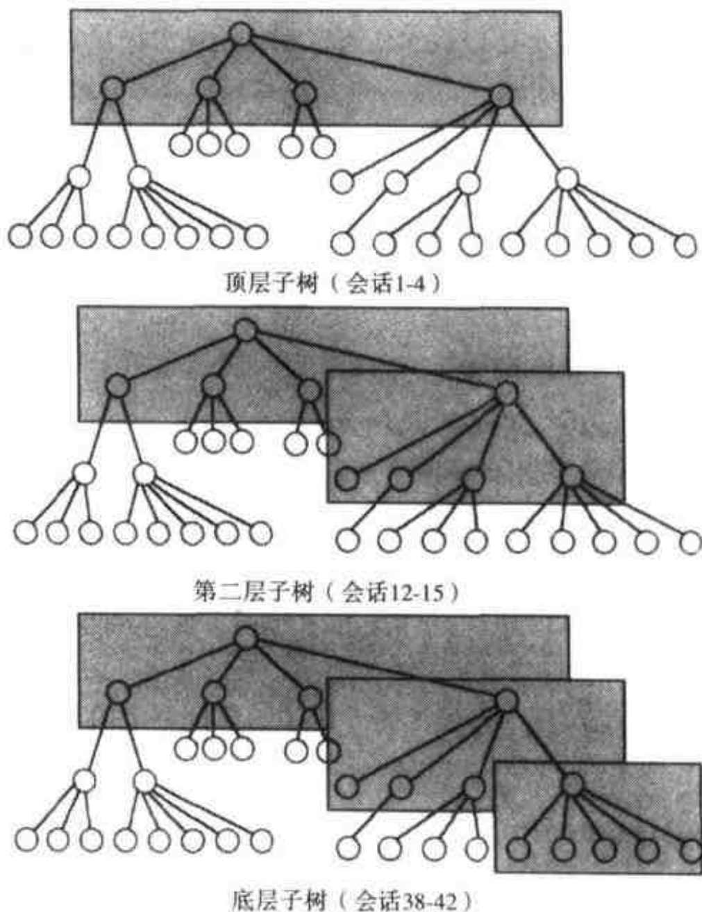
图13-3 自顶向下集成
