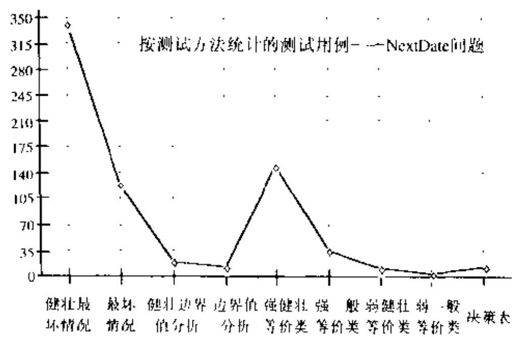
图8-4 NextDate问题的测试用例趋势线
