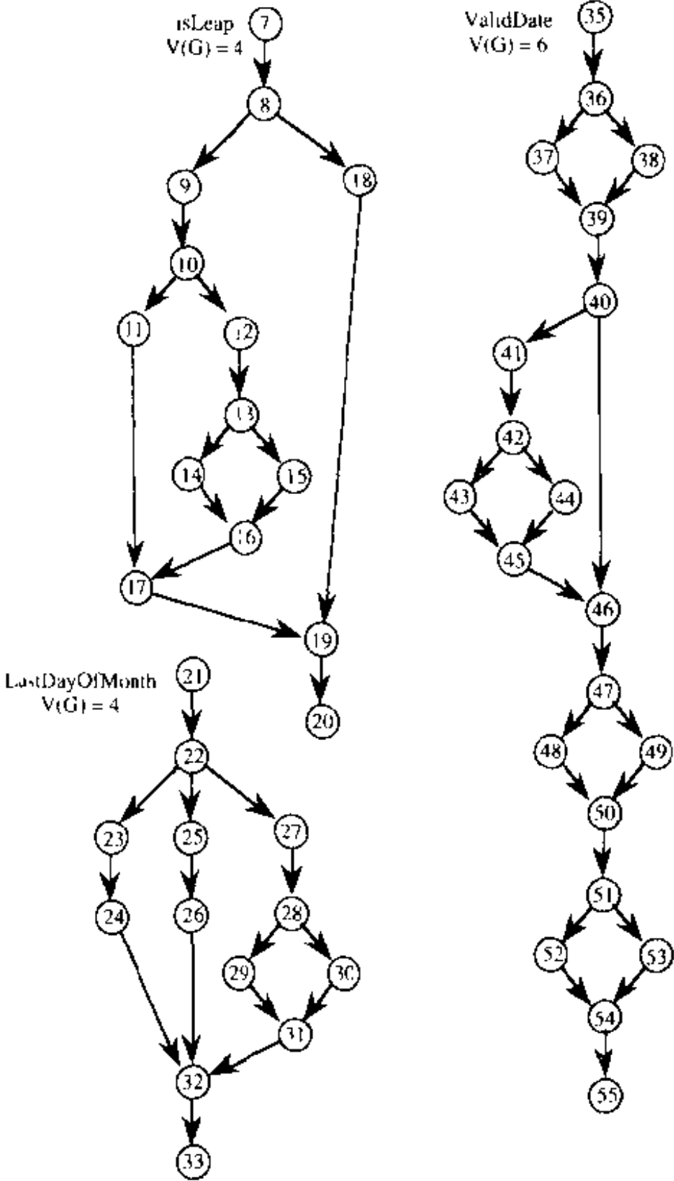
图13-14 低层单元
