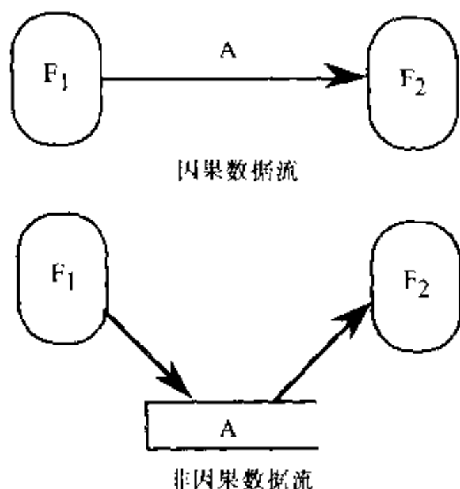
图13-10 数据静止
