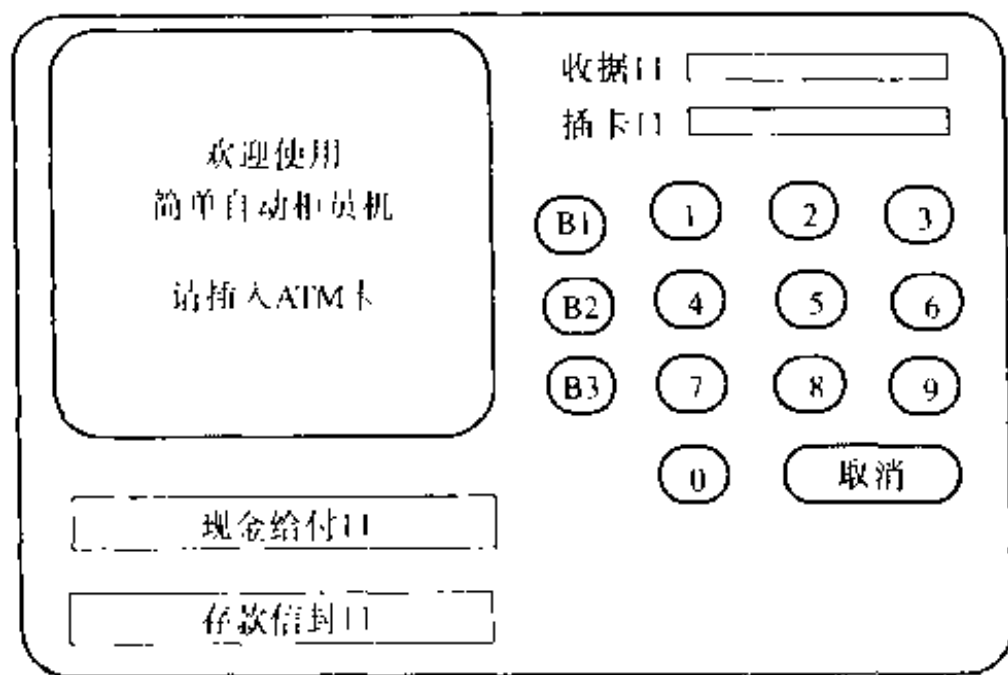
图2-3 SATM终端
