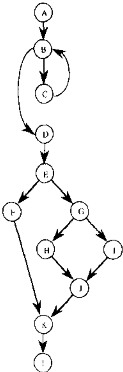
图10-2 佣金问题的DD-路径图
