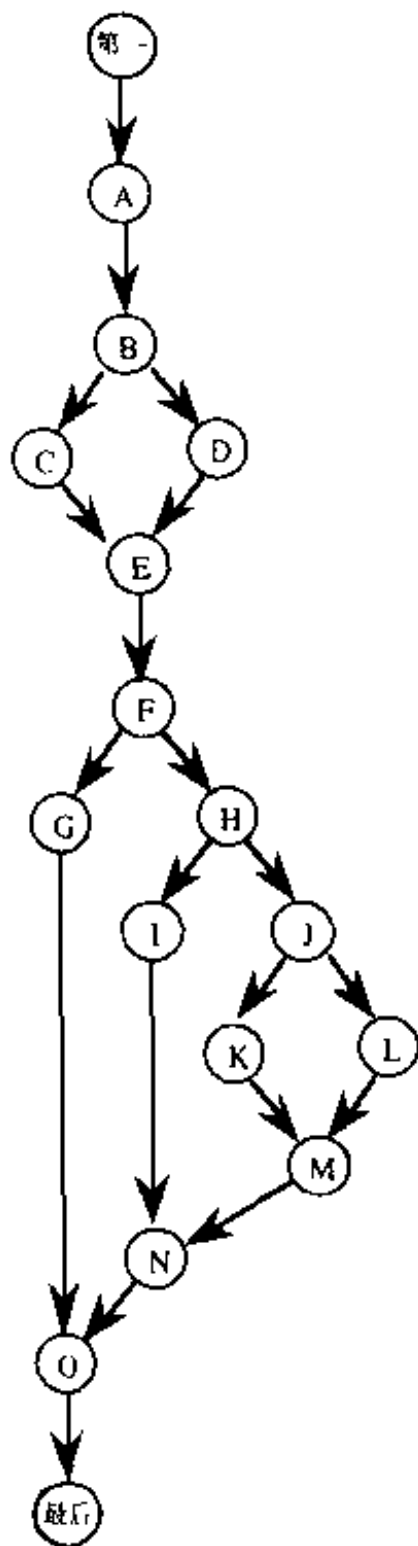
图9-4 三角形程序的DD-路径图
