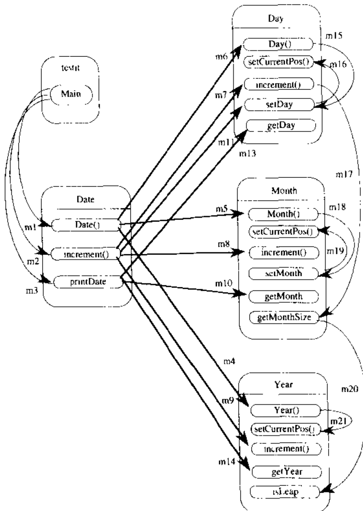
图18-3 o-oCalendar中的消息
