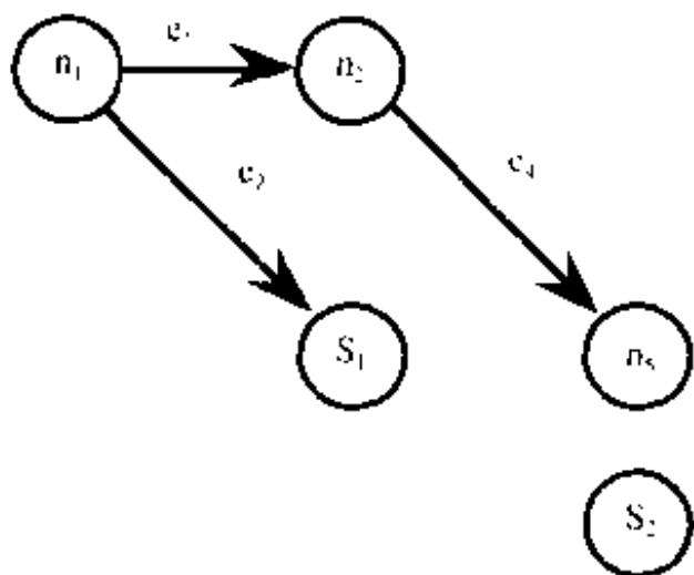
图4-4 图4-3所示有向图的压缩图
