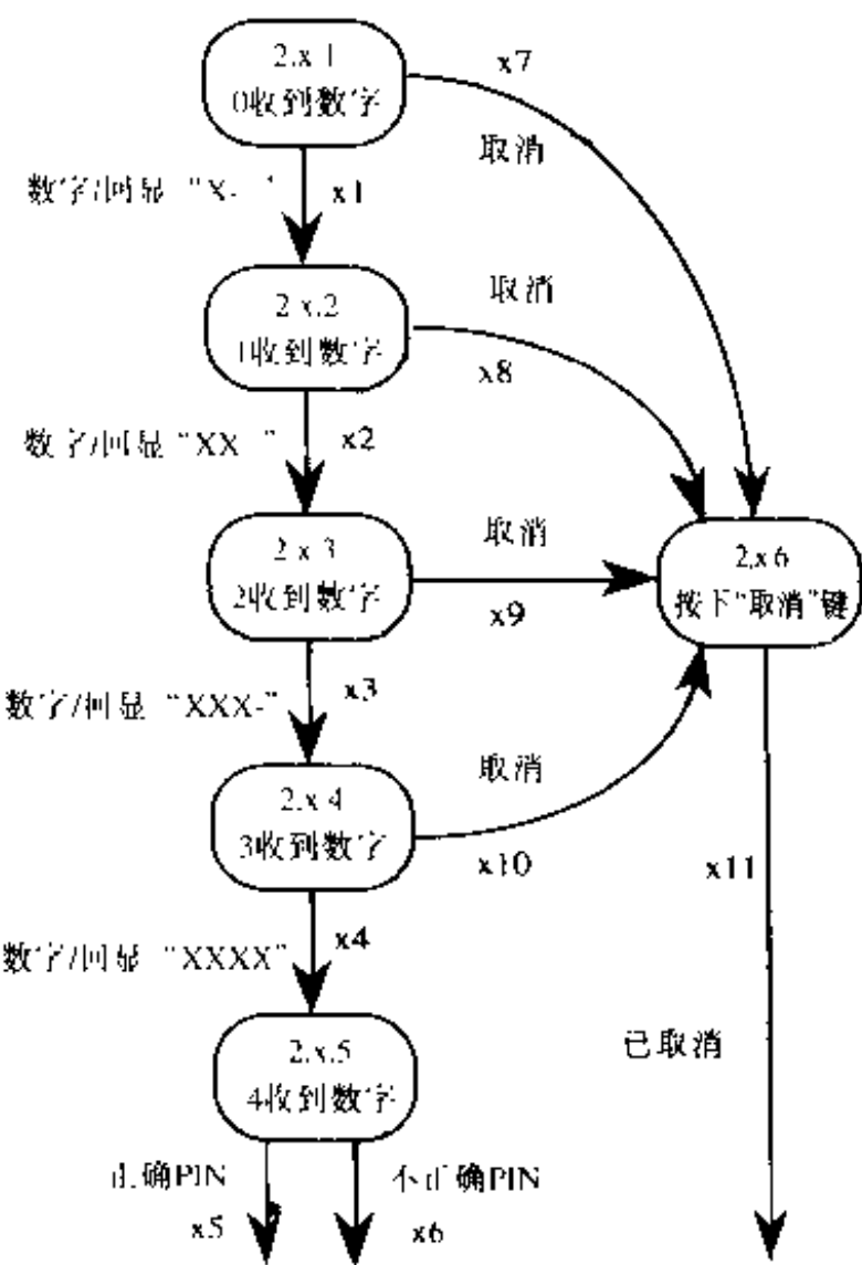
图14-7 “PIN输入尝试”有限状态机
