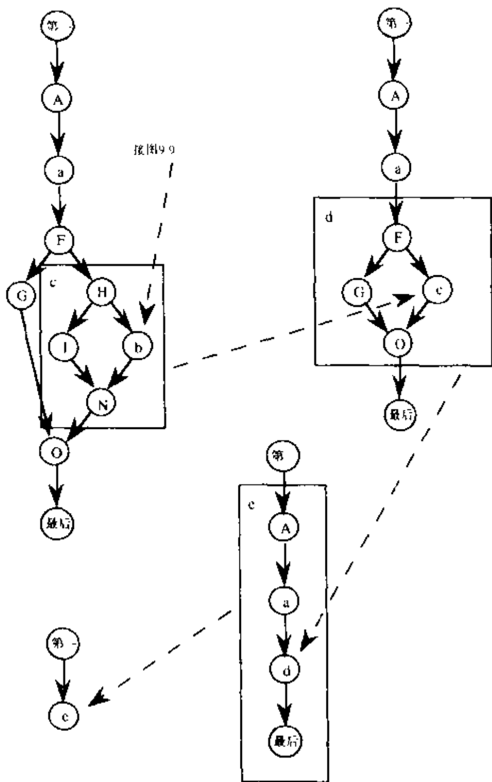
图9-10 根据结构化程序设计构造压缩(续)
