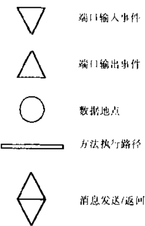
图18-6 EMDPN的符号
