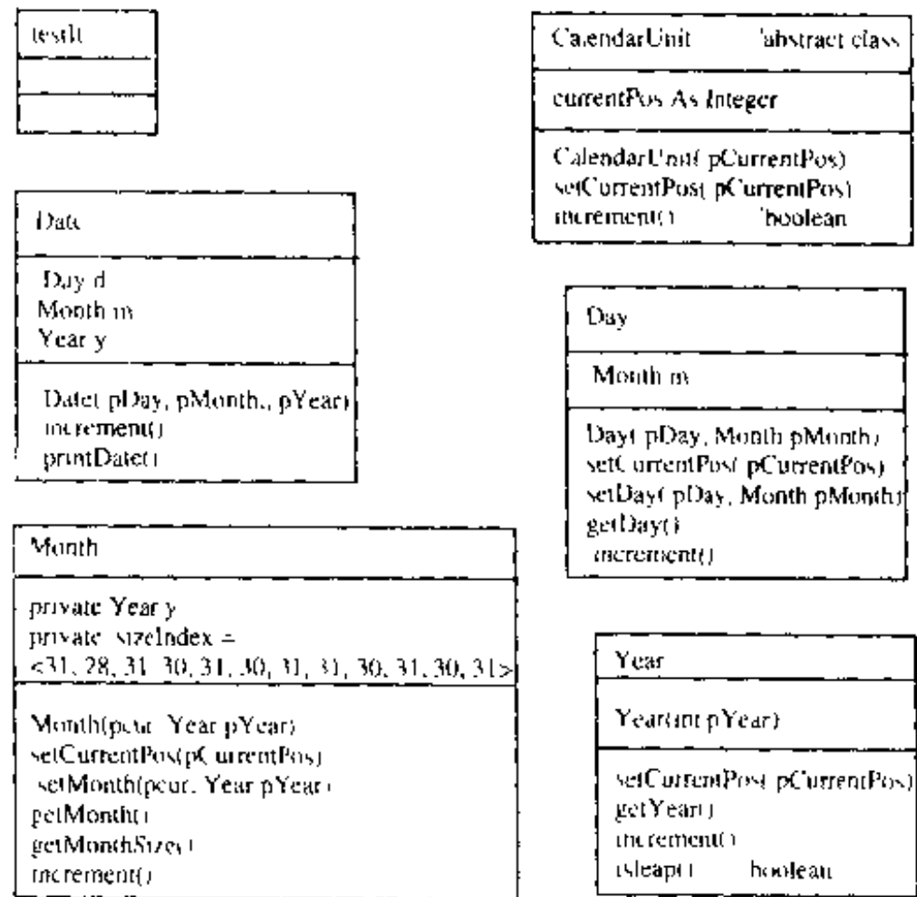
图16-4 o-oCalendar中的类
