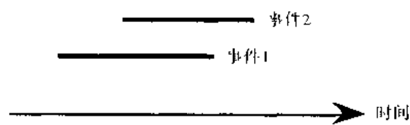
图15-1 重叠的事件
