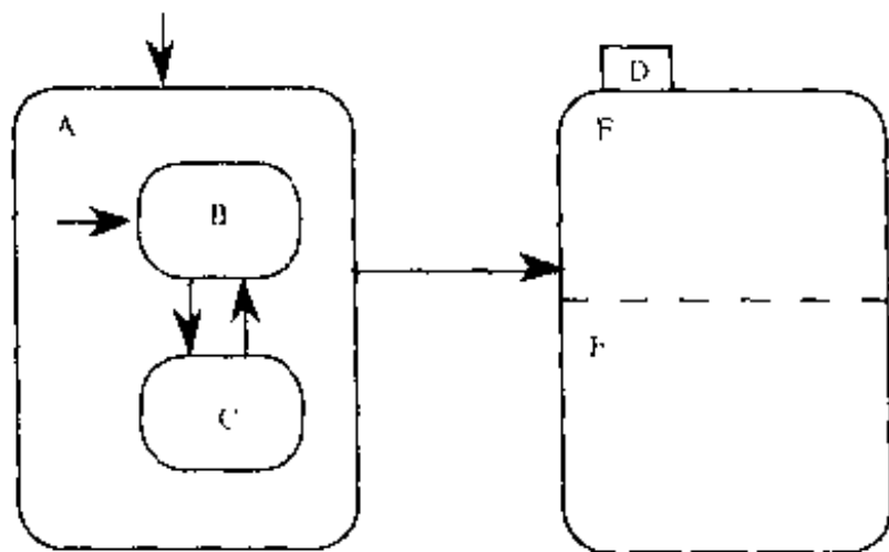
图4-14 并发状态
