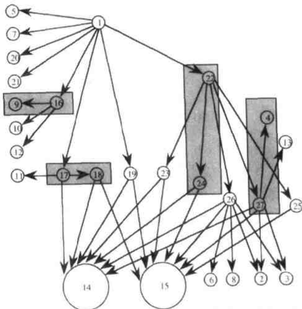
图13-6 成对集成
