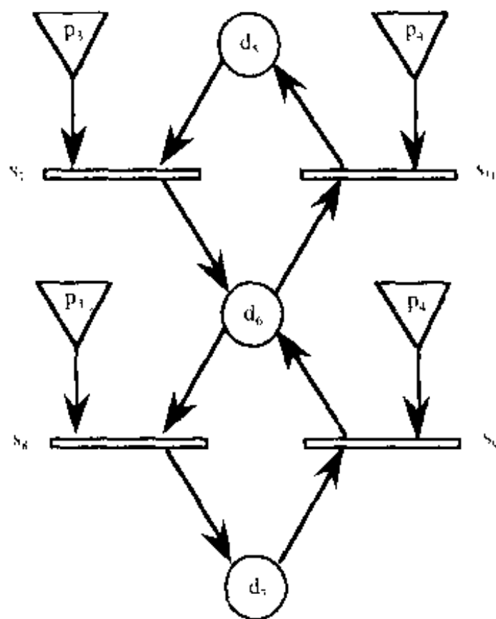
图4-10 EDPN
