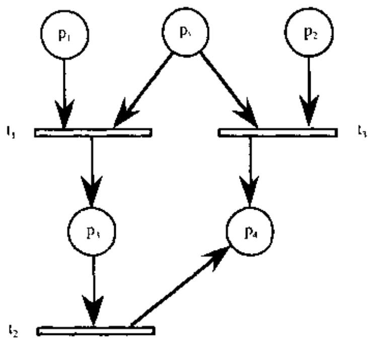
图4-7 Petri网
