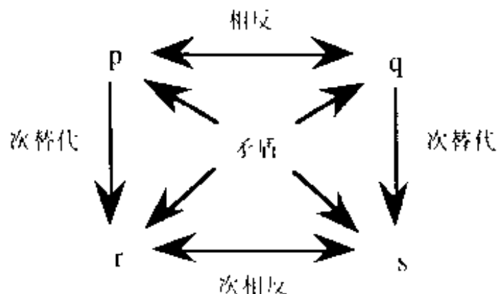
图15-3 相反正方形
