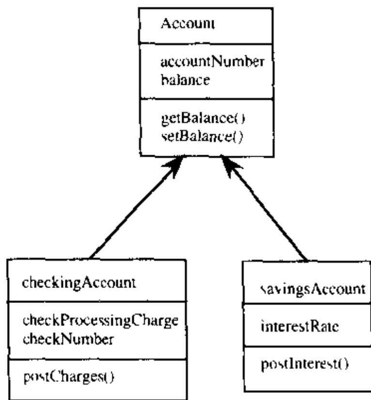
图16-2 类继承
