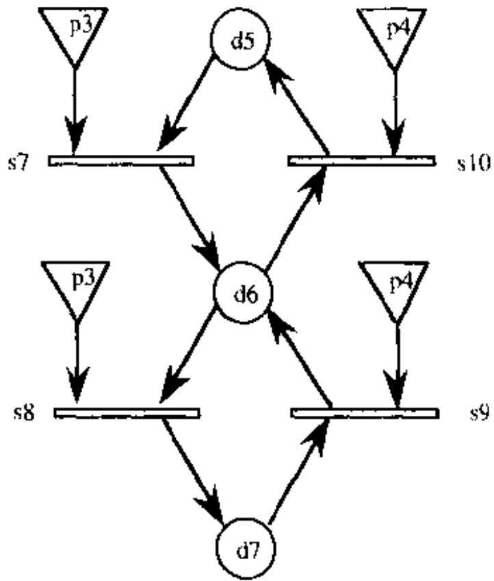
图15-10 刻度盘EDPN
