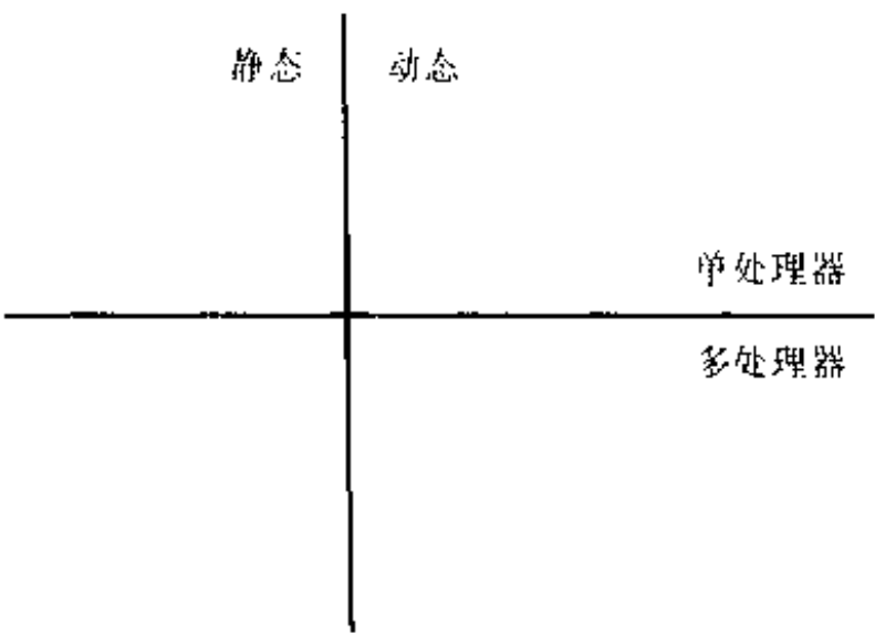
图15-2 交互类型
