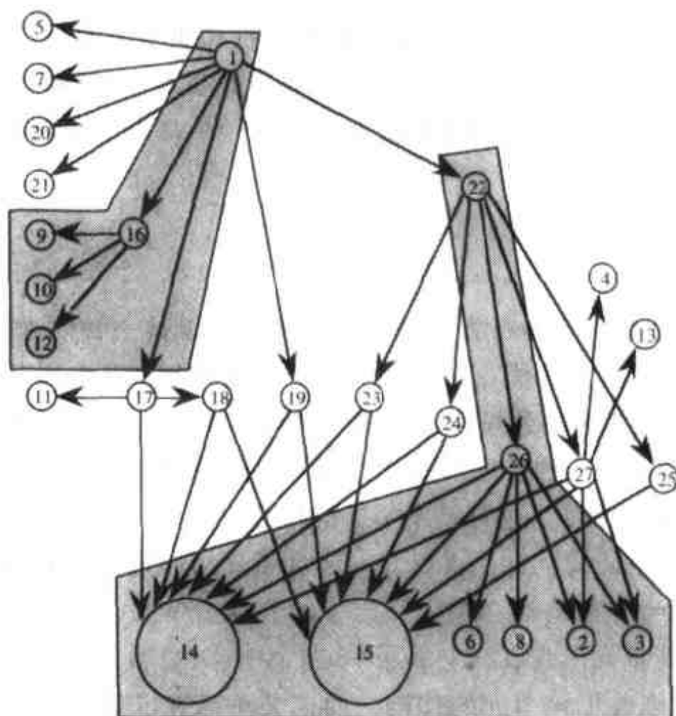
图13-7 相邻集成
