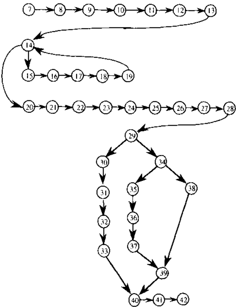
图10-1 佣金问题的程序图
